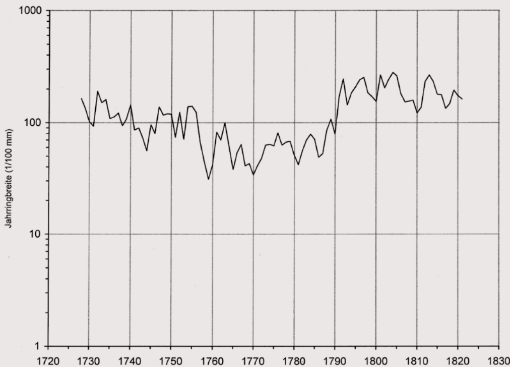
Abb. 3 Kurve der Jahrringbreiten nach der Einpassung in die Eichen-Standard-Chronologie. Grafik: Jahrringlabor Hofmann, Nürtingen.
