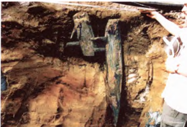
Abb. 16: In den sandigen Untergrund gerammter Eichenpfahl als Teil der Brückenkonstruktion an der heutigen Maxbrücke (Foto: AAF).
